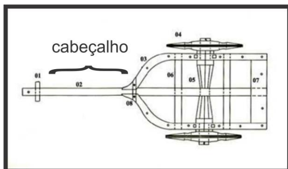
Figura XXI – Ilustração do cabeçalho no carro de boi.
